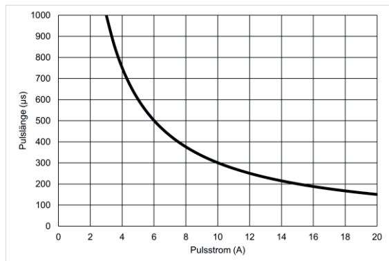
Pulslänge in Abhängigkeit vom Pulsstrom
