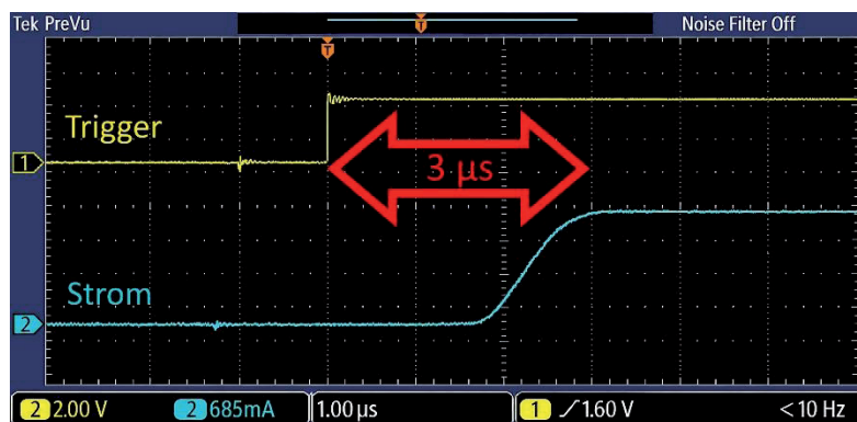
Pulsverzögerungen von nur 3 µs
